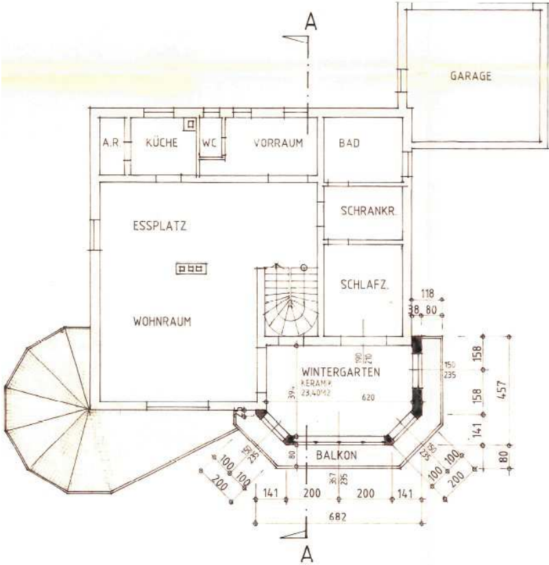
ERDGESCHOSS
