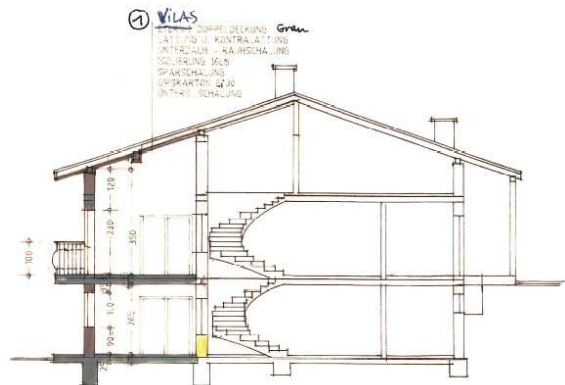
SCHNITT A-A
