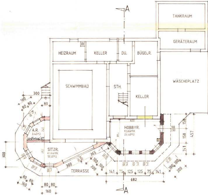
UNTERGESCHOSS
